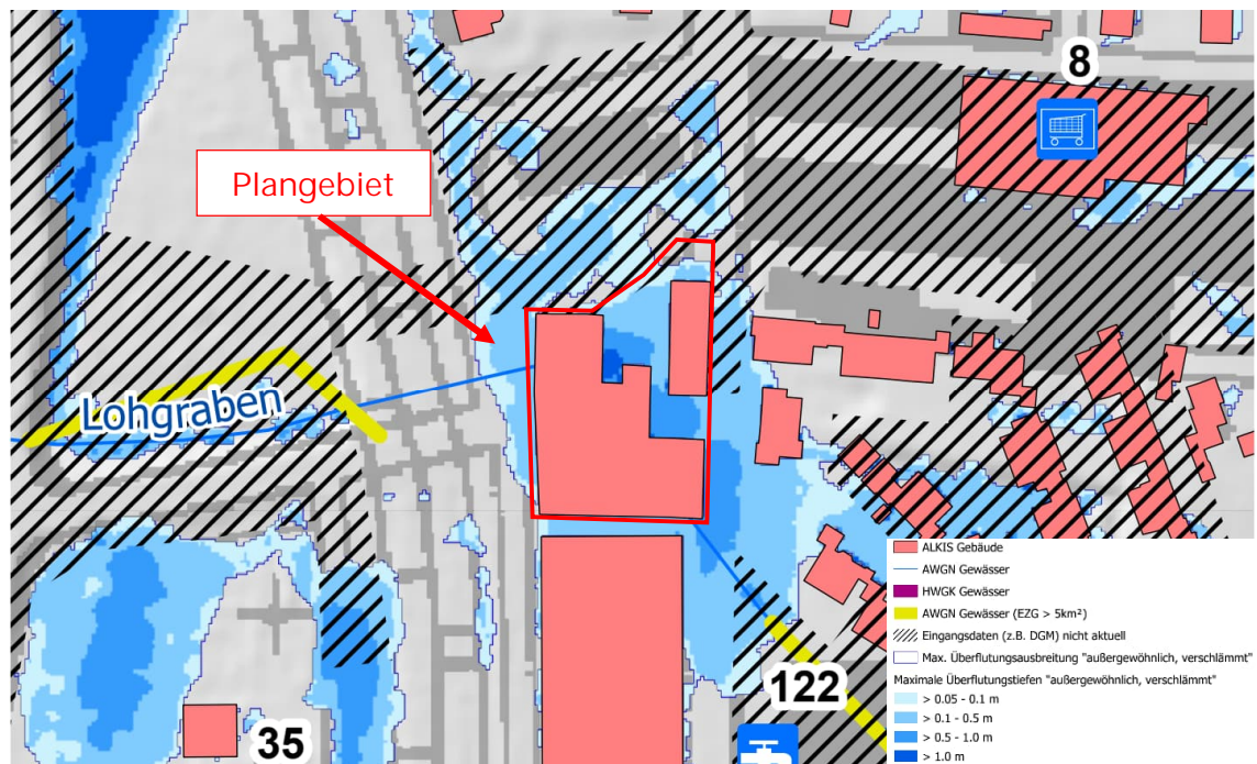
Abb. 9: Starkregenrisikokarte Stadt Gundelsheim (Quelle: BIT Ingenieure AG)
